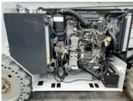
Motore diesel Yanmar 3 cilindri 18 kW
